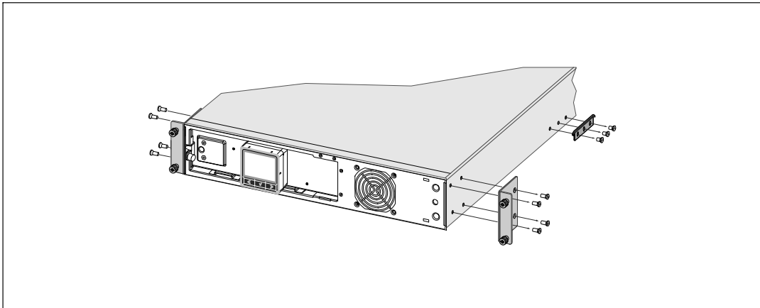
그림 19. 장착 브래킷 및 뒷면 고정(hold-down) 브래킷 분리하기
