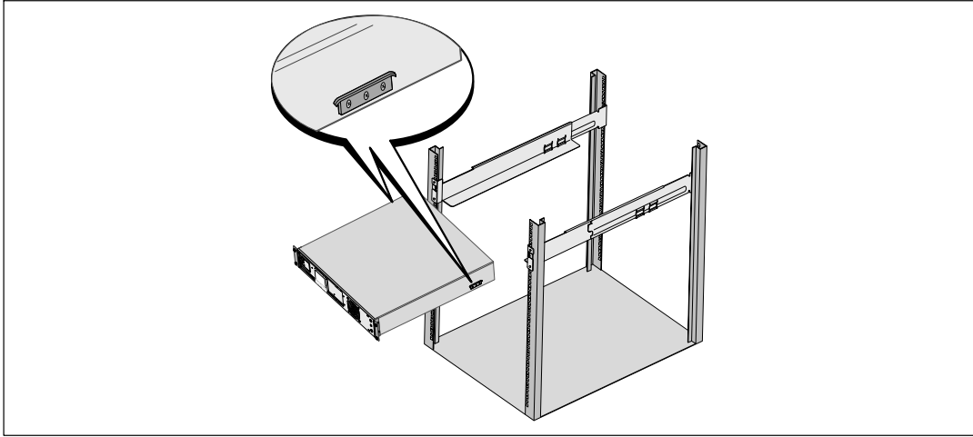
그림 15. 캐비닛 설치하기
