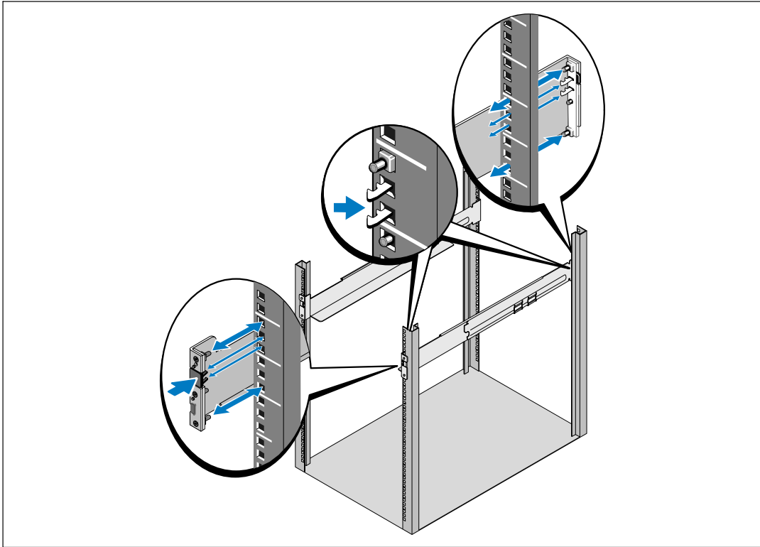
그림 14. 레일 설치하기
